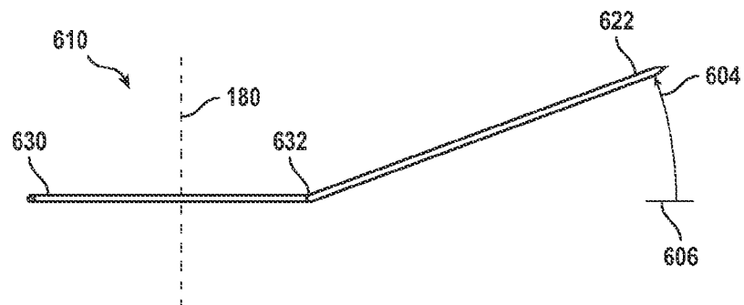
VIEW A-A FIG. 6B
