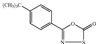
5-(4-tert-Butyl-phenyl)-[1,3,4]oxathiazol-2-one
