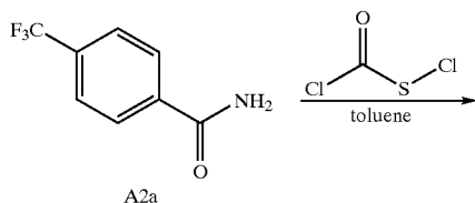
Scheme A2
