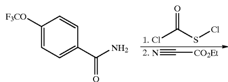
Scheme D2
