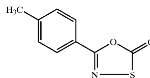
5-p-Tolyl-[1,3,4]oxathiazol-2-one
