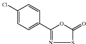
5-(4-Chloro-phenyl)-[1,3,4]oxathiazol-2-one
