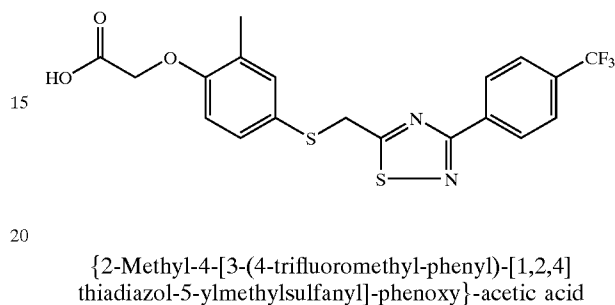
Scheme A1
