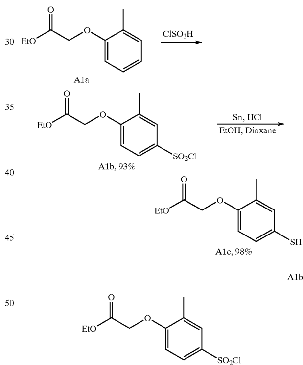
Scheme A1
