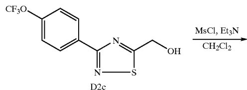
Scheme E2
