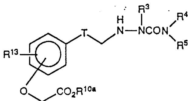
(Ia-6)
