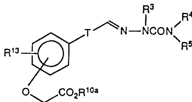
(Ia-5)
