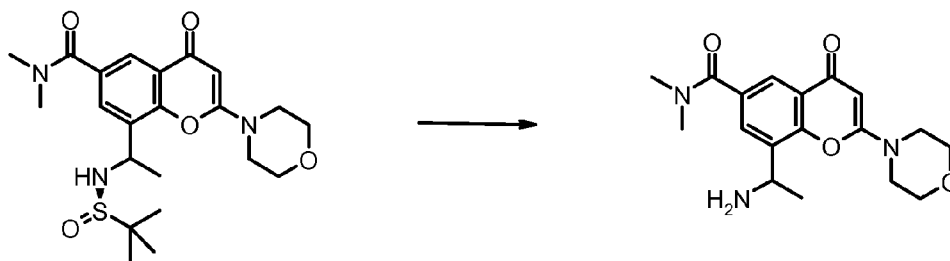
Single enantiomer
