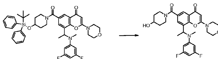
enantiomer 2
