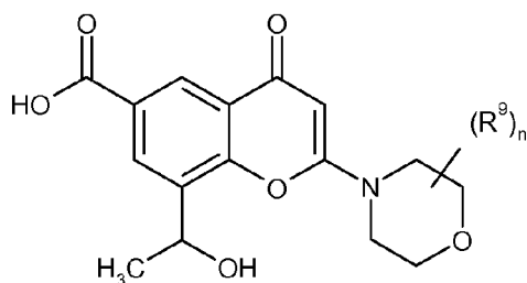
XVa
