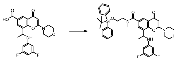
enantiomer 1
