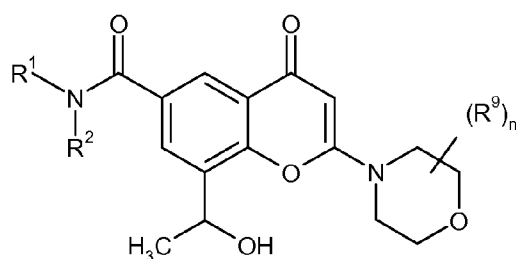
XV
