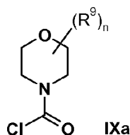
IXa
