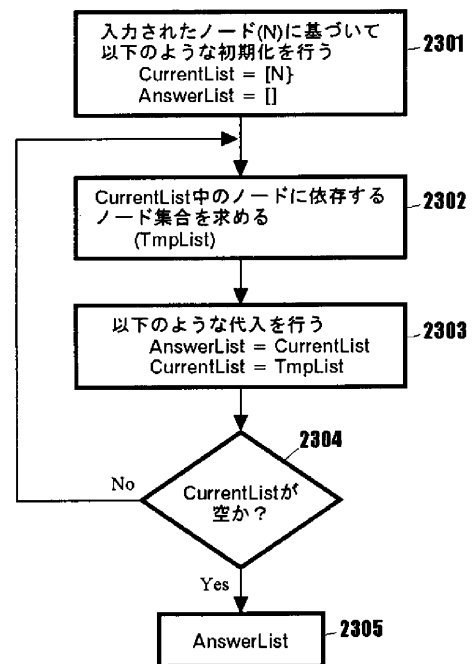
依存関係にあるノードを見つける処理
