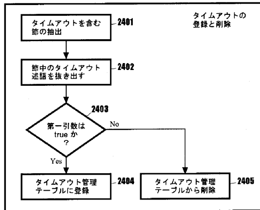
タイムアウトの登録と削除の詳細
