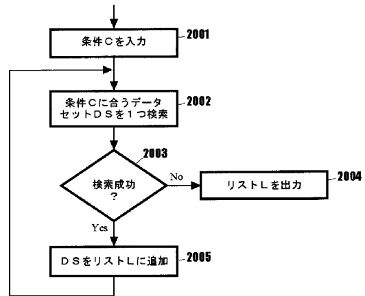
すべての要素を見つけるための処理
