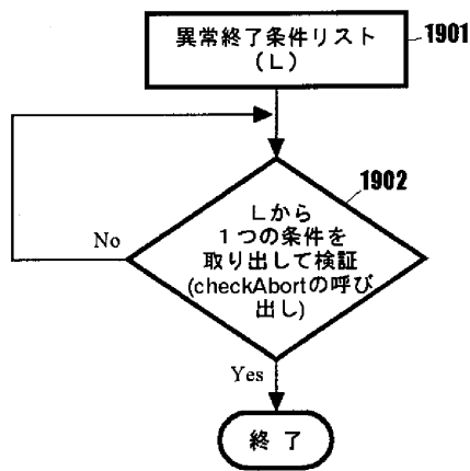
異常終了の判定
