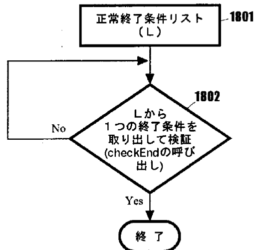
正常終了の判定
