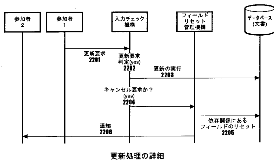
更新処理の詳細
