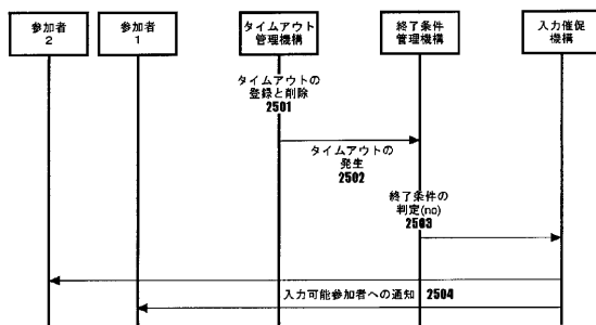
タイムアウトの登録と発生後の処理
