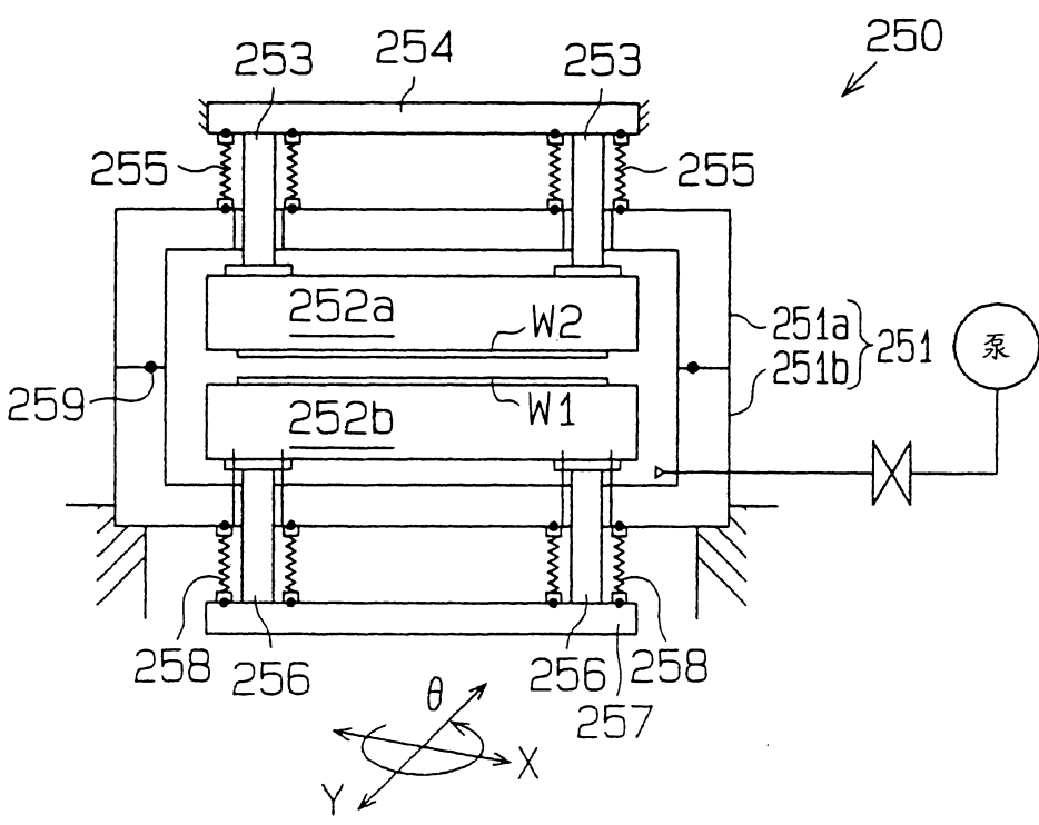
對於第31圖之習知例的概略構成圖
