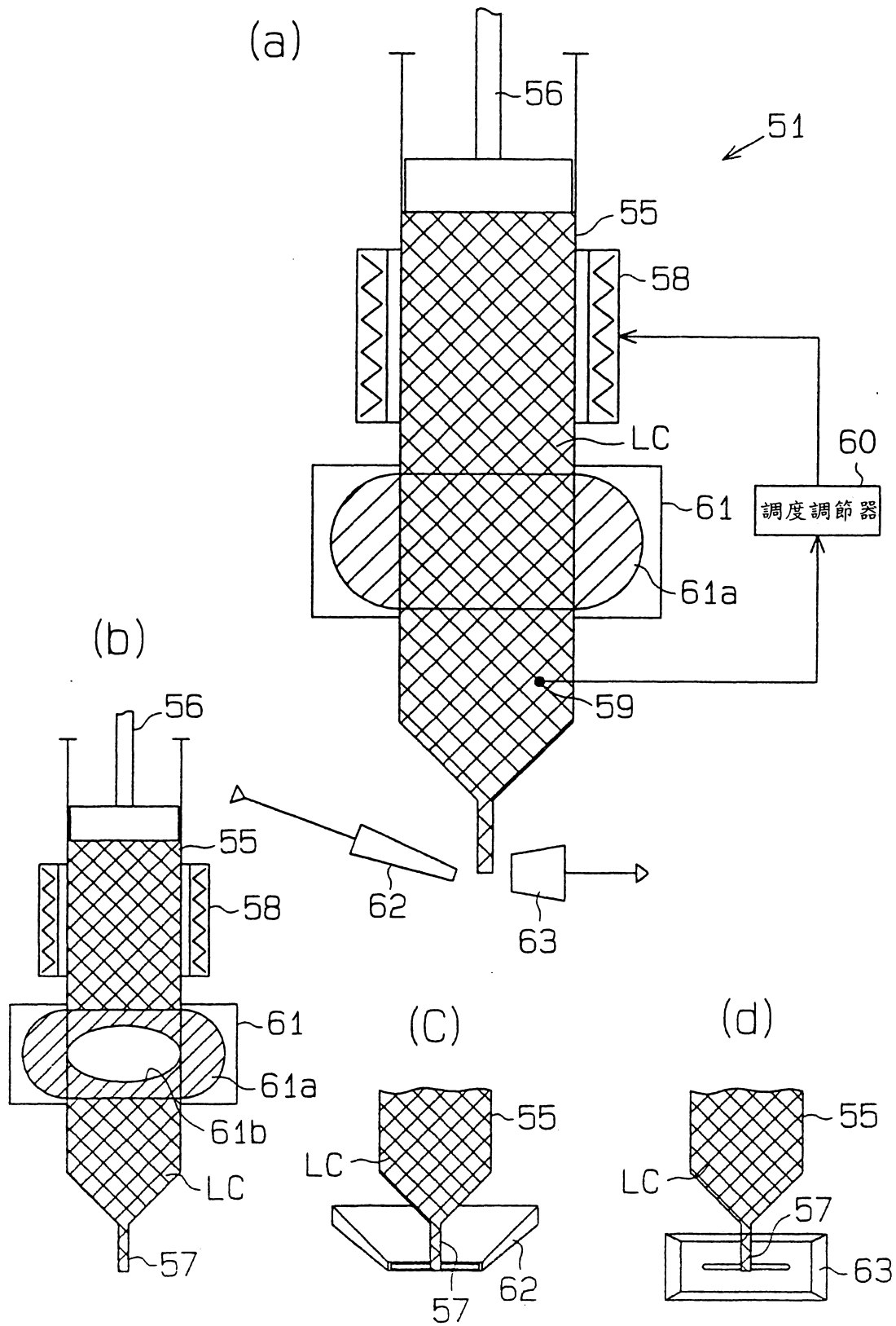
給料器之說明圖
