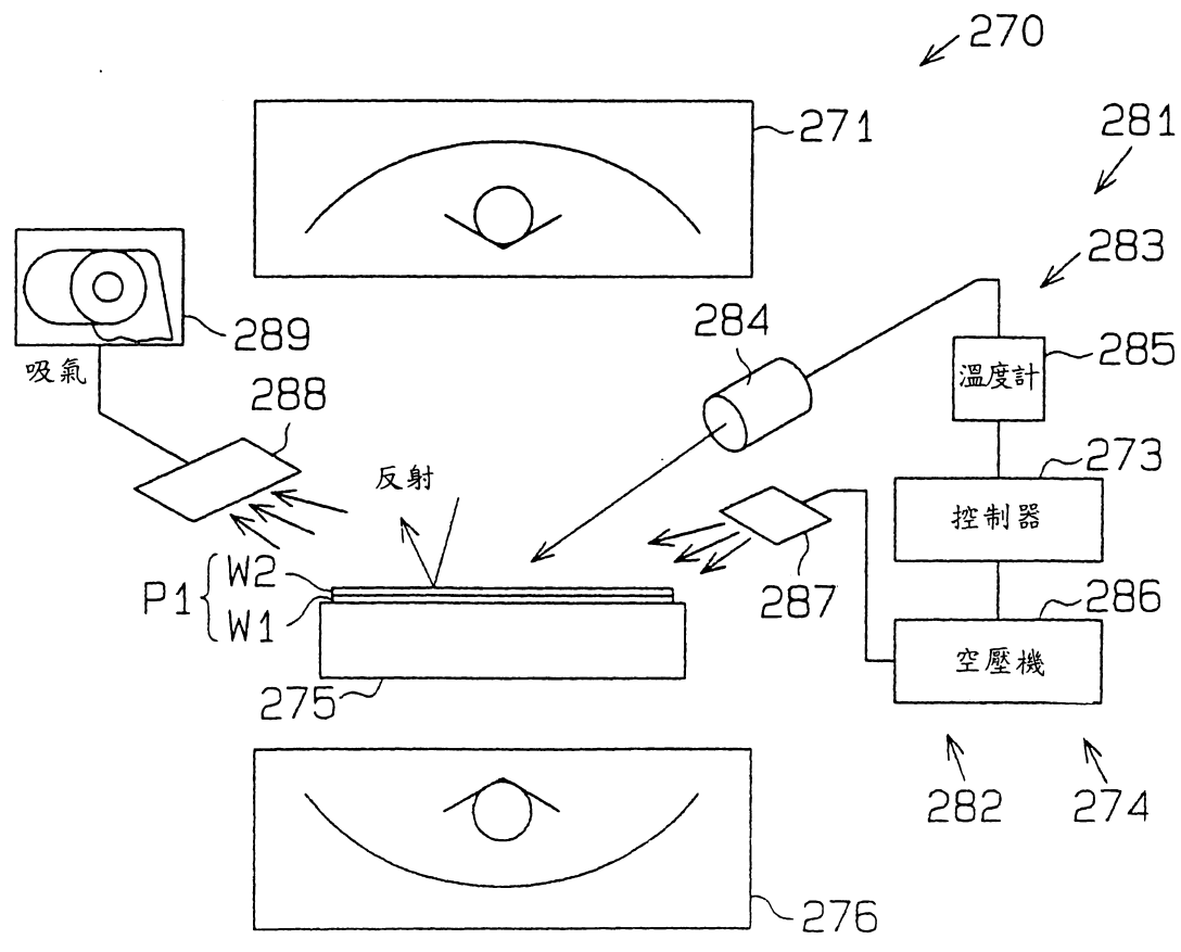
其他密封材硬化裝置之概略構成圖
