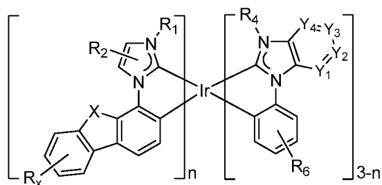
Formula VI.
