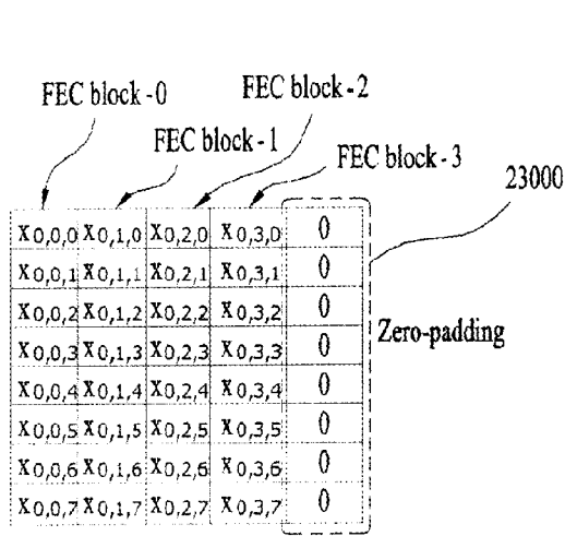
[TI FEC blocks]
