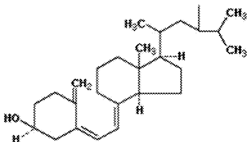
Vitamin D-2
