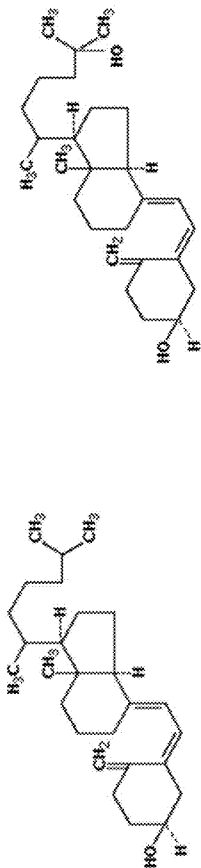
Vitamin D-3
