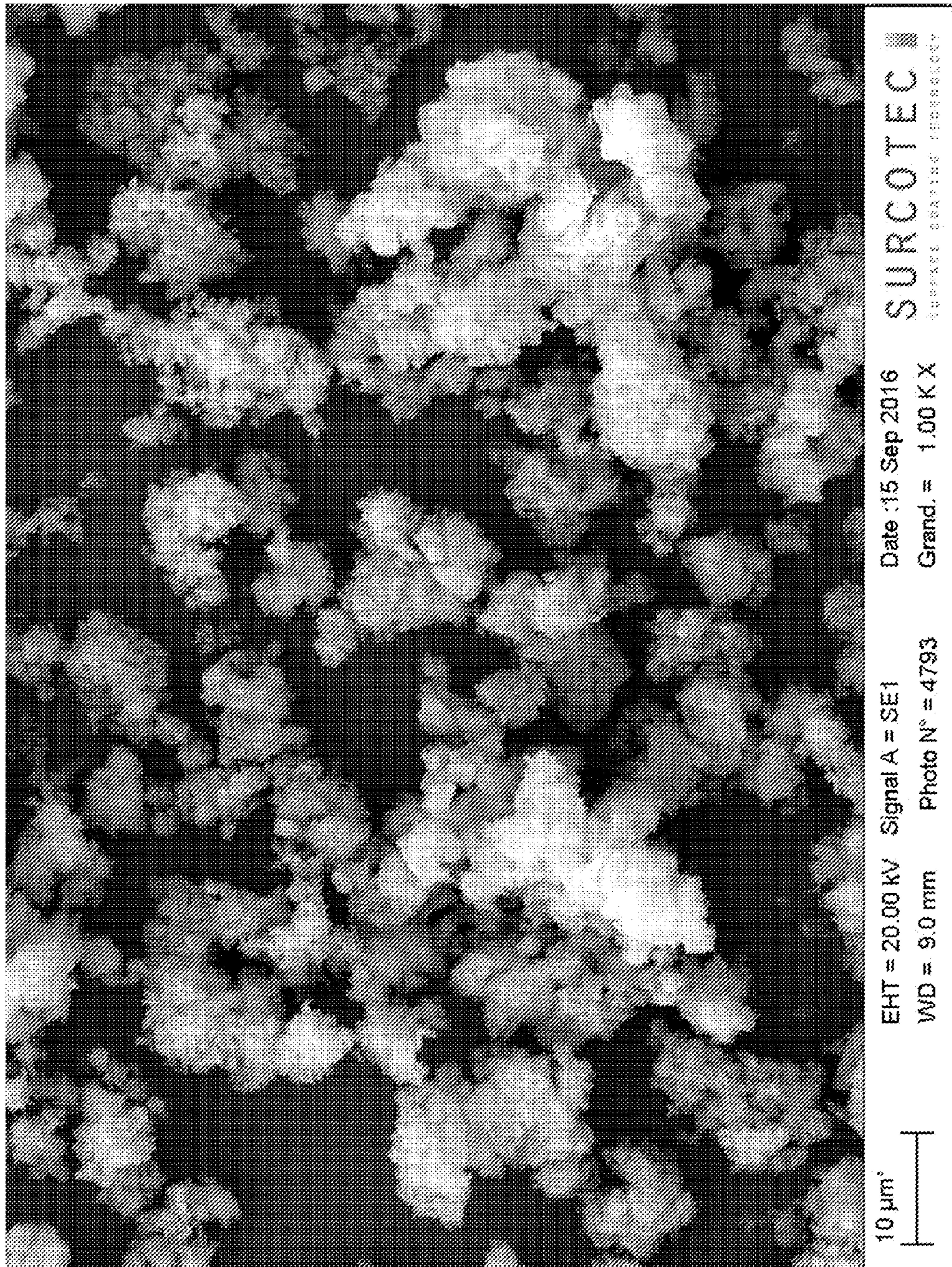
Figure 8 : Cliché MEB des cristaux de diglycéroxyde de calcium fait avec les billes Silibeads 2mm (échantillon 241.1)
