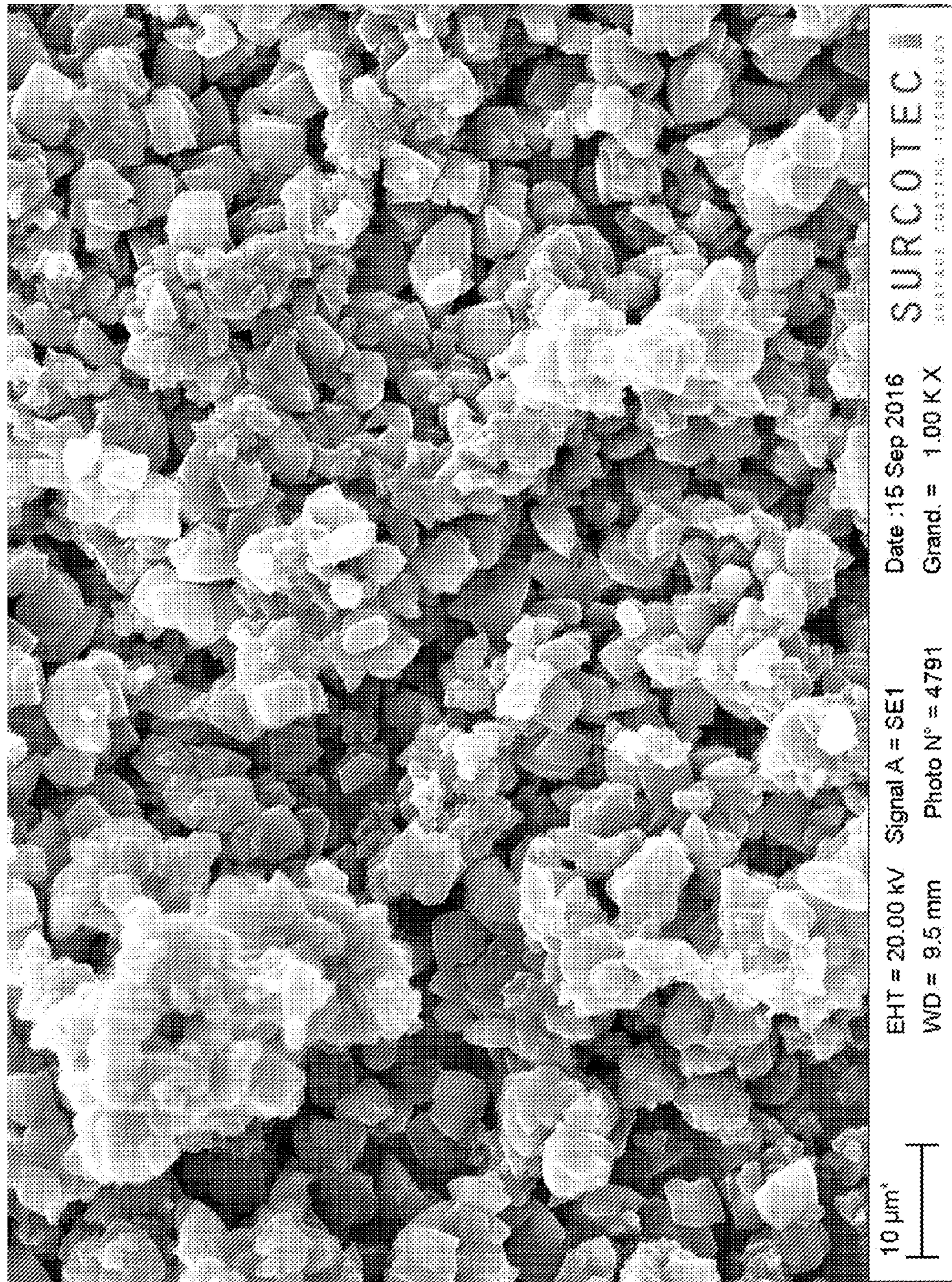
Figure 6 : Cliché MEB des cristaux de diglycéroxyde de calcium faits avec les billes Zirmill 0.5 mm
