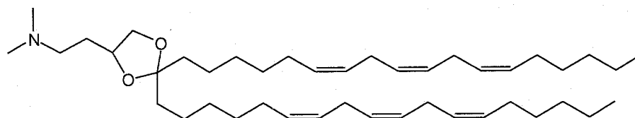
\gamma -DLen-C2K-DMA
