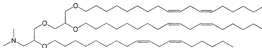
TLinDMA
