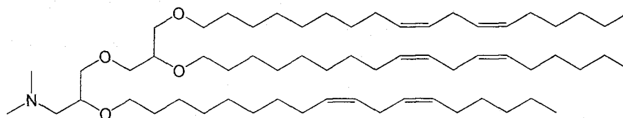
TLinDMA
