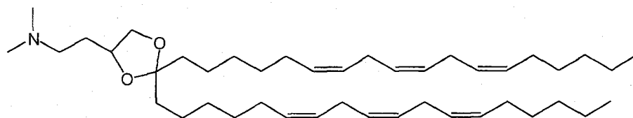
\gamma -DLen-C2K-DMA
