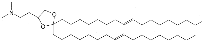
DHep-C2K-DMA
