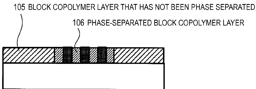
FIG. 1B ANNEALING
