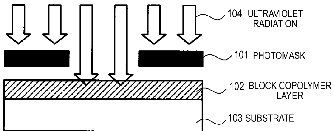
FIG. 1A EXPOSURE
