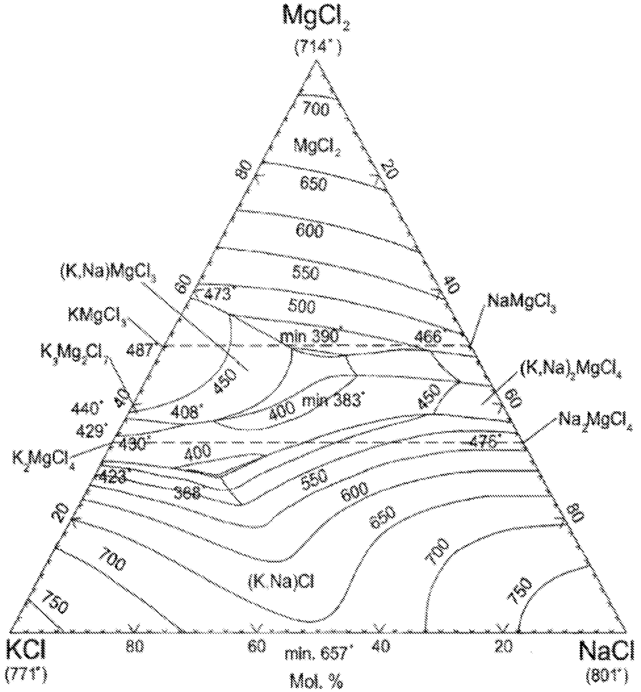
Figura 1 (Técnica anterior)
