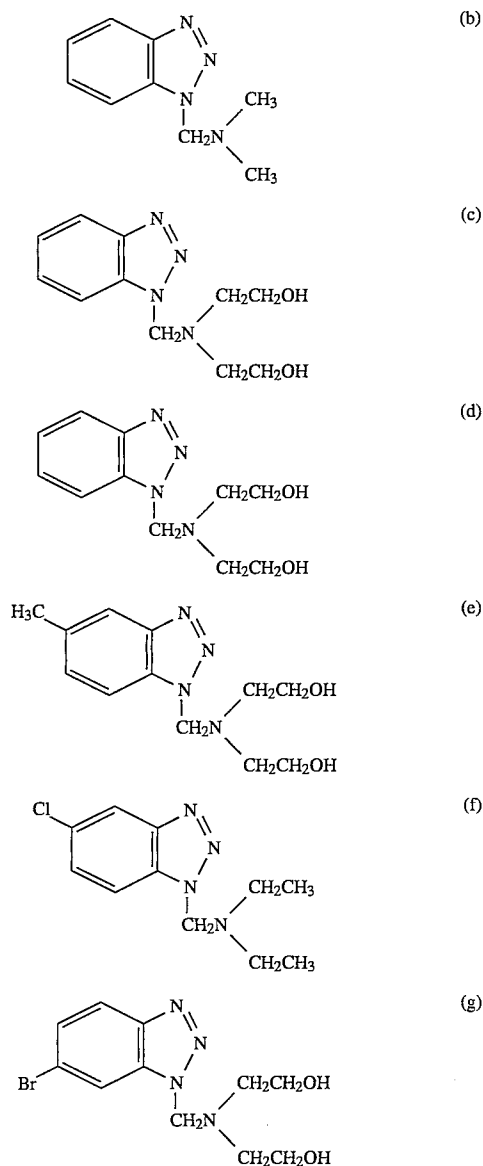
Benztriazole compounds
