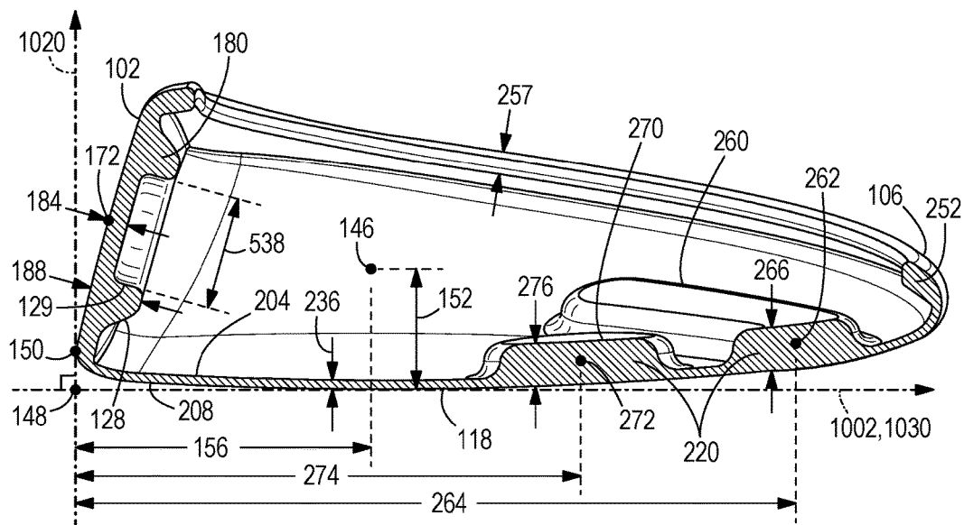
FIG. 6 Section A-A
