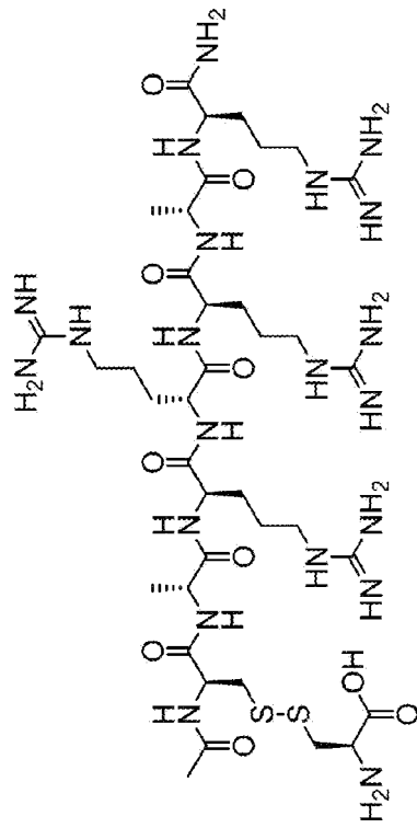
Ac-D-Cys(L-Cys-OH)-D-Ala-D-Arg-D-Arg-D-Arg-D-Arg-D-Ala-D-Arg-NH 2
