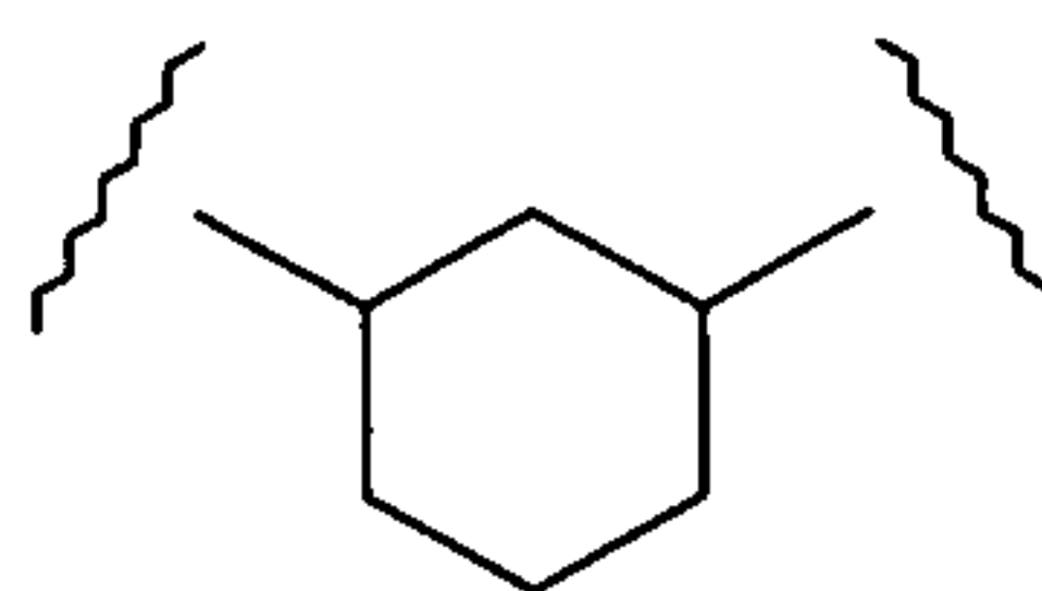
cyclohexane-1,3-di-yl
