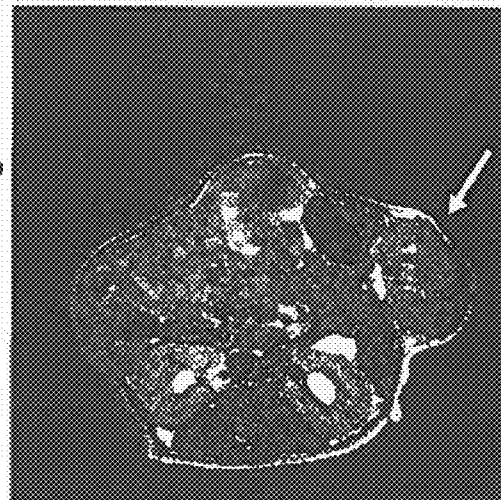
scL-HK-Mag
