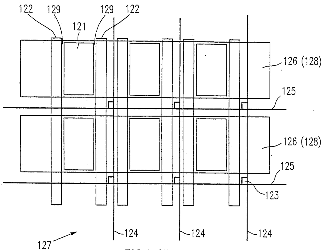
TOP VIEW FIG. 12A
