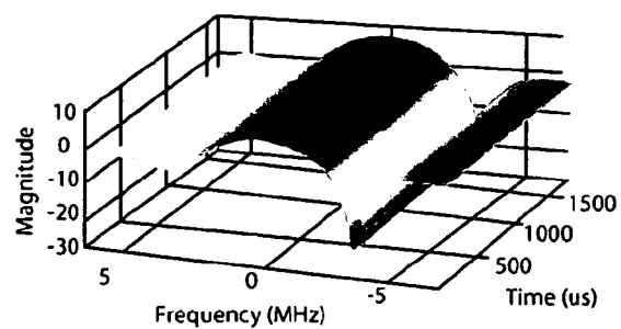
(b) Magnitude
