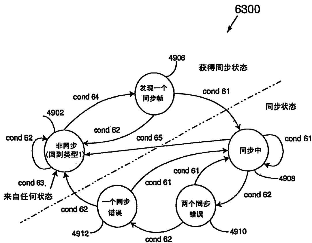
图 63 cond 61 = 子帧报头数据包 & 处于帧边界的正确 CRC, 帧长度 > 0 cond 62 = 非同步模式或帧边界处的错误 CRC cond 63 = 接收链路关闭数据包 cond 64 = 发现同步模式 cond 65 = 唯一字不正确
