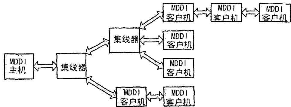
集线器与串级链组合
