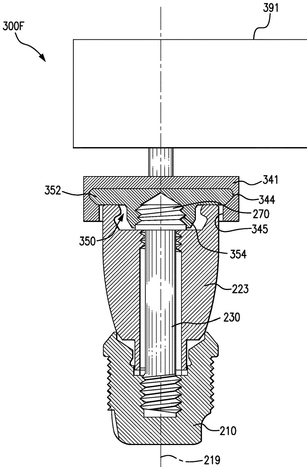
FIG. 3F
