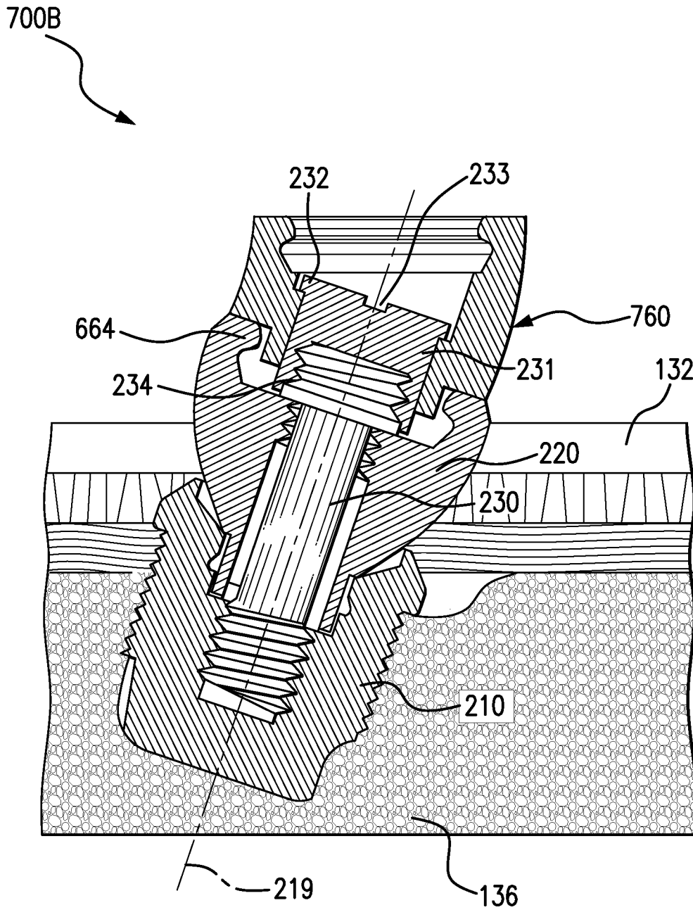
FIG. 7B
