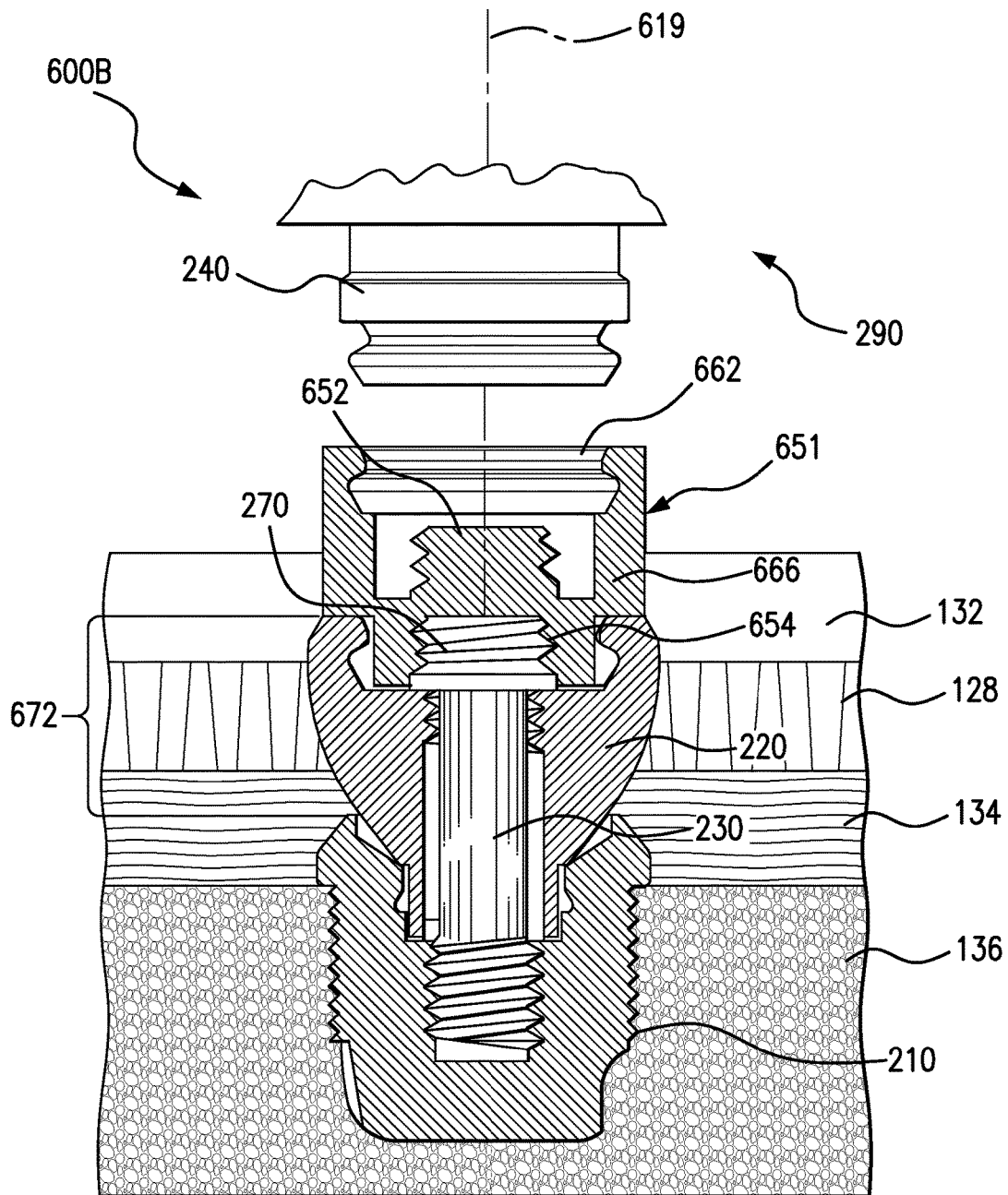
FIG. 6B
