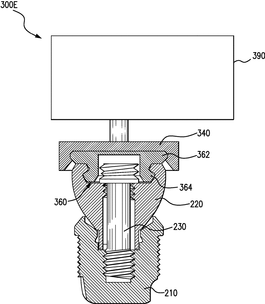
FIG. 3E
