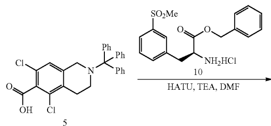
Scheme E3
