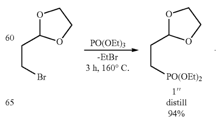
Scheme E4B
