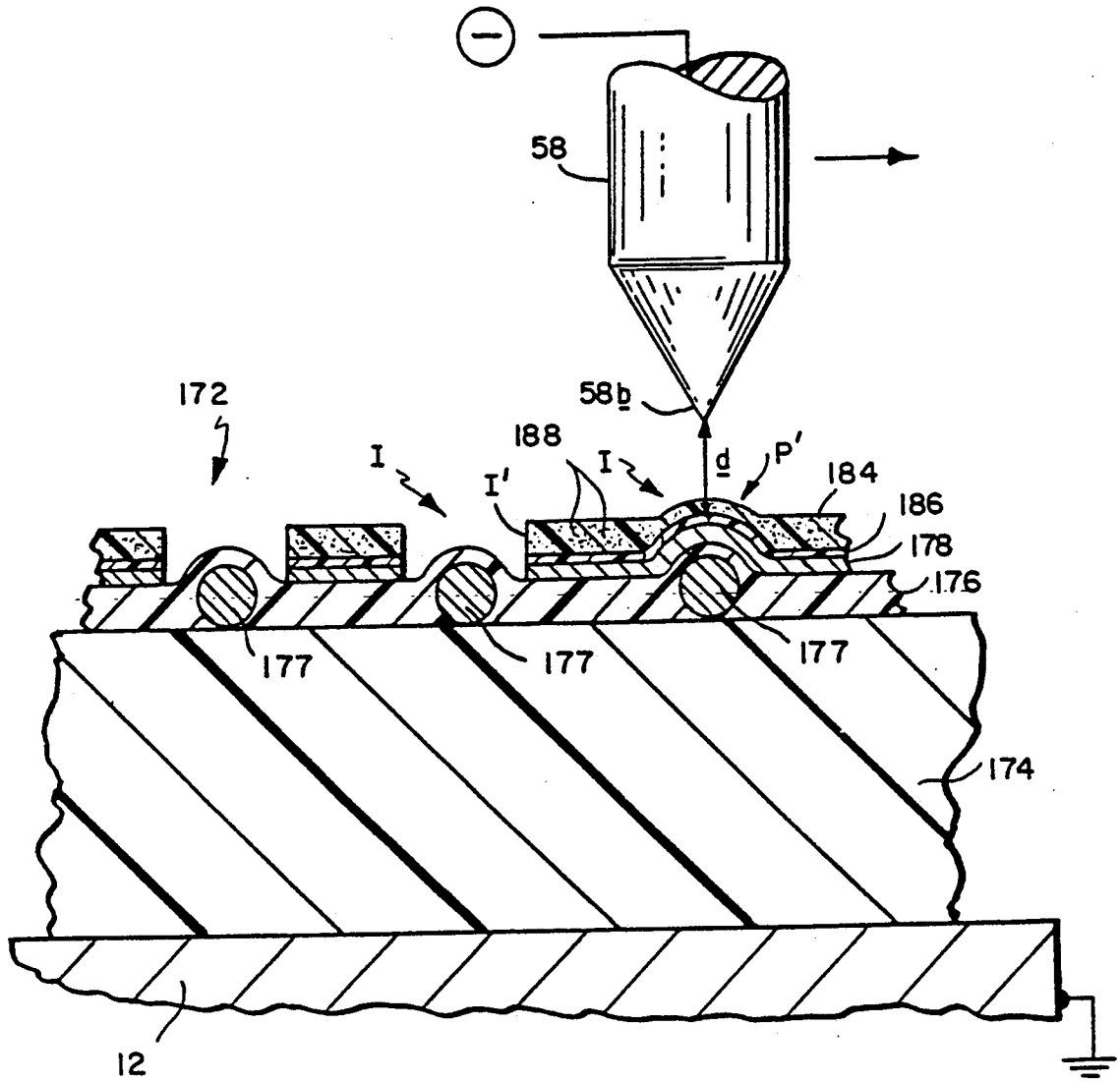
FIG. 4F
