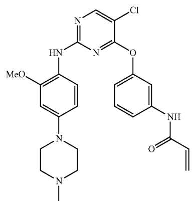
WZ4002
