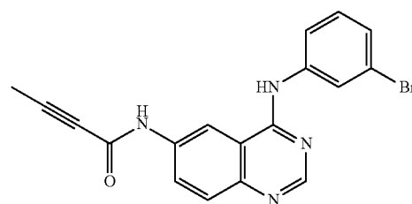
CL-387785
