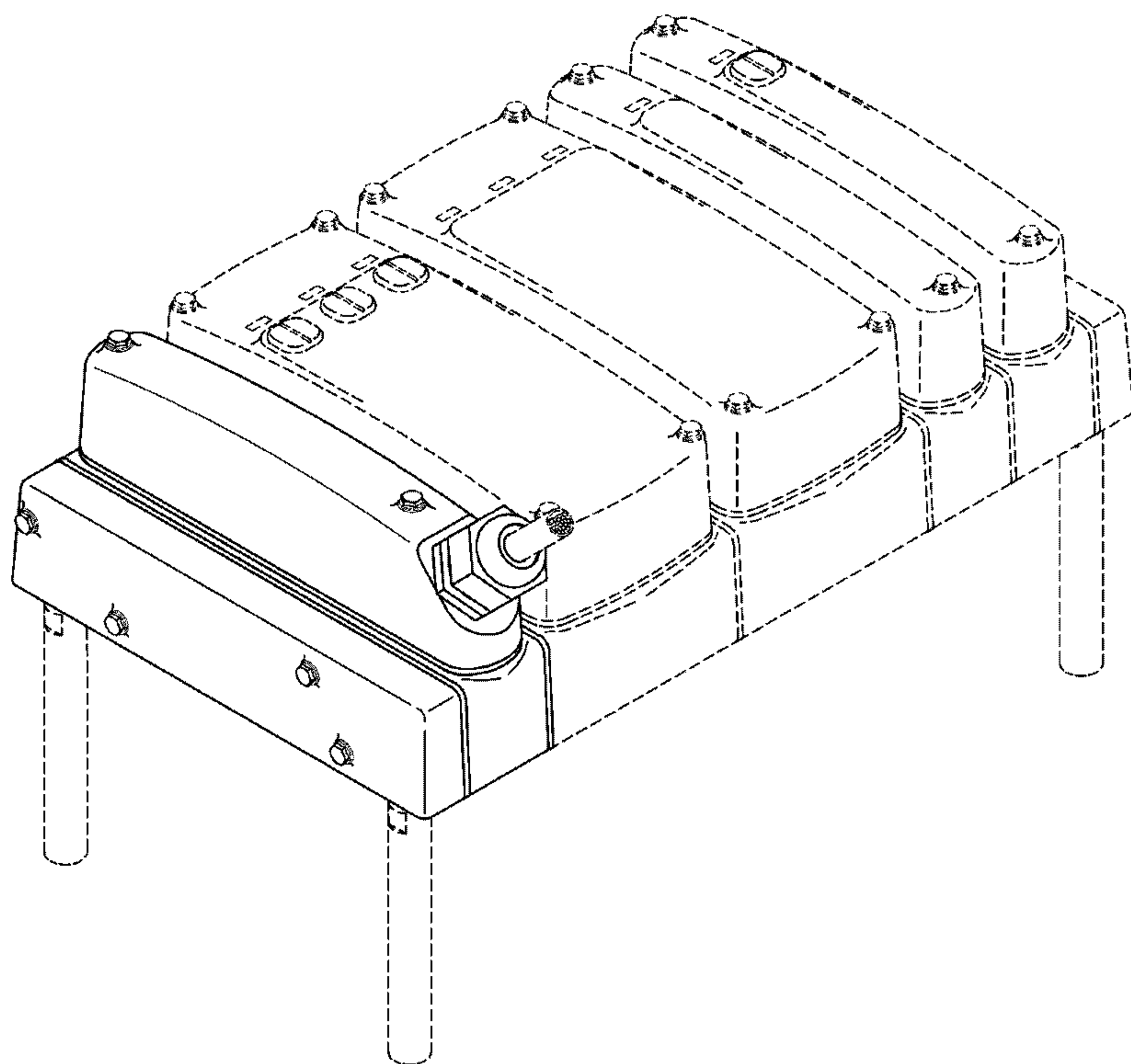
【立體圖 1】
