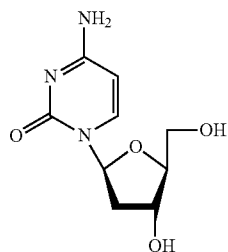
\beta -L-dC
