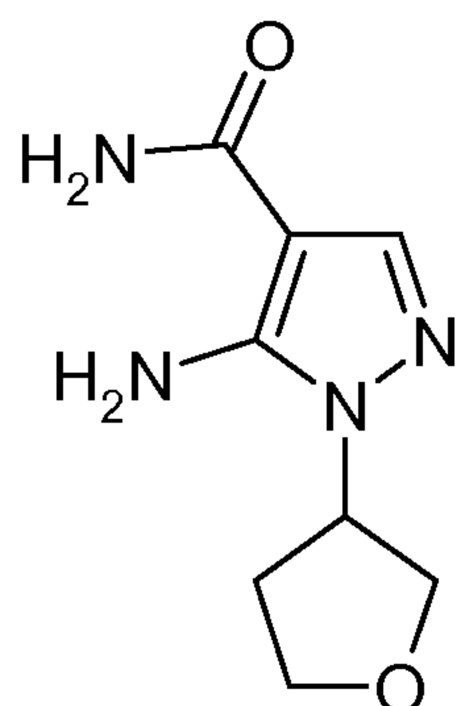
Enantiomer B
