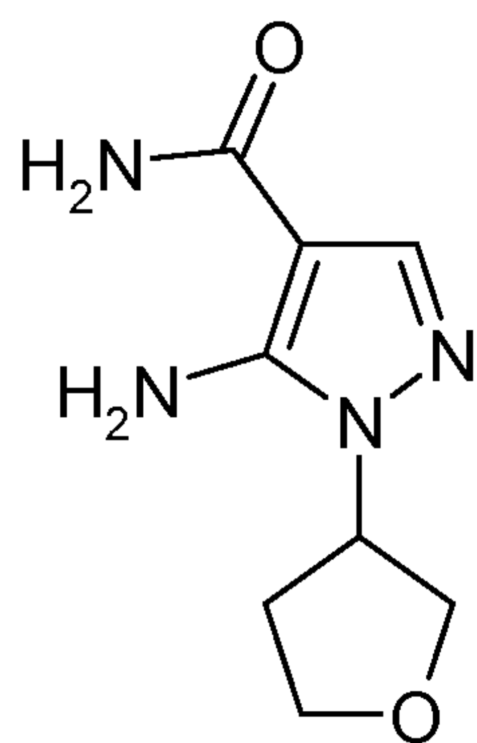
Enantiomer A
