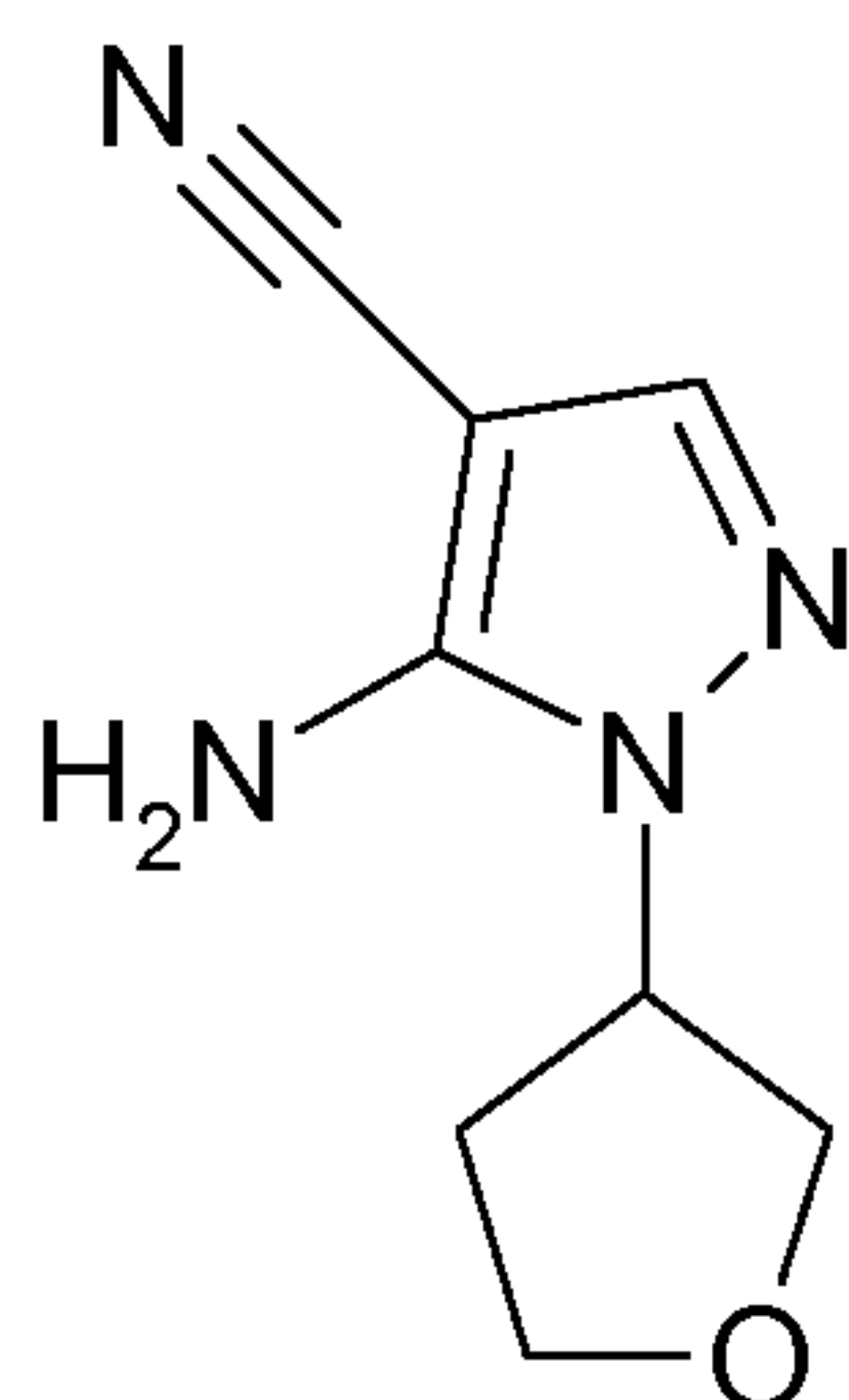
Enantiomer B
