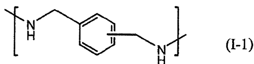
[Chemical 3]
