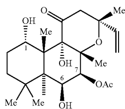
Forskolin
