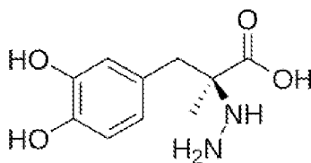
carbidopa
