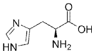
L-histidine
