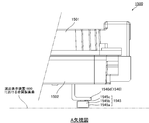
A矢視図
