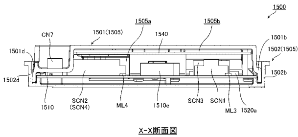
X-X断面図
