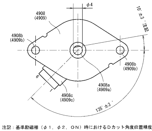
(a) Dカット角度位置
