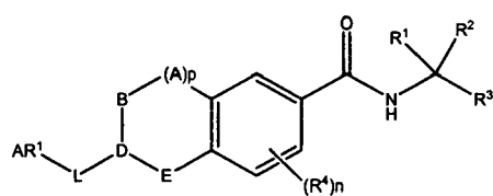
Fomula I
