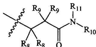
Formula VII-b
