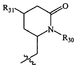
X-a
