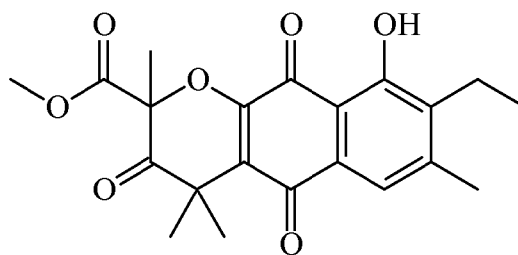
Annulin B
