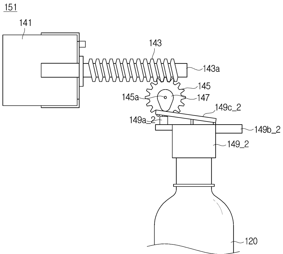
FIG. 9A
