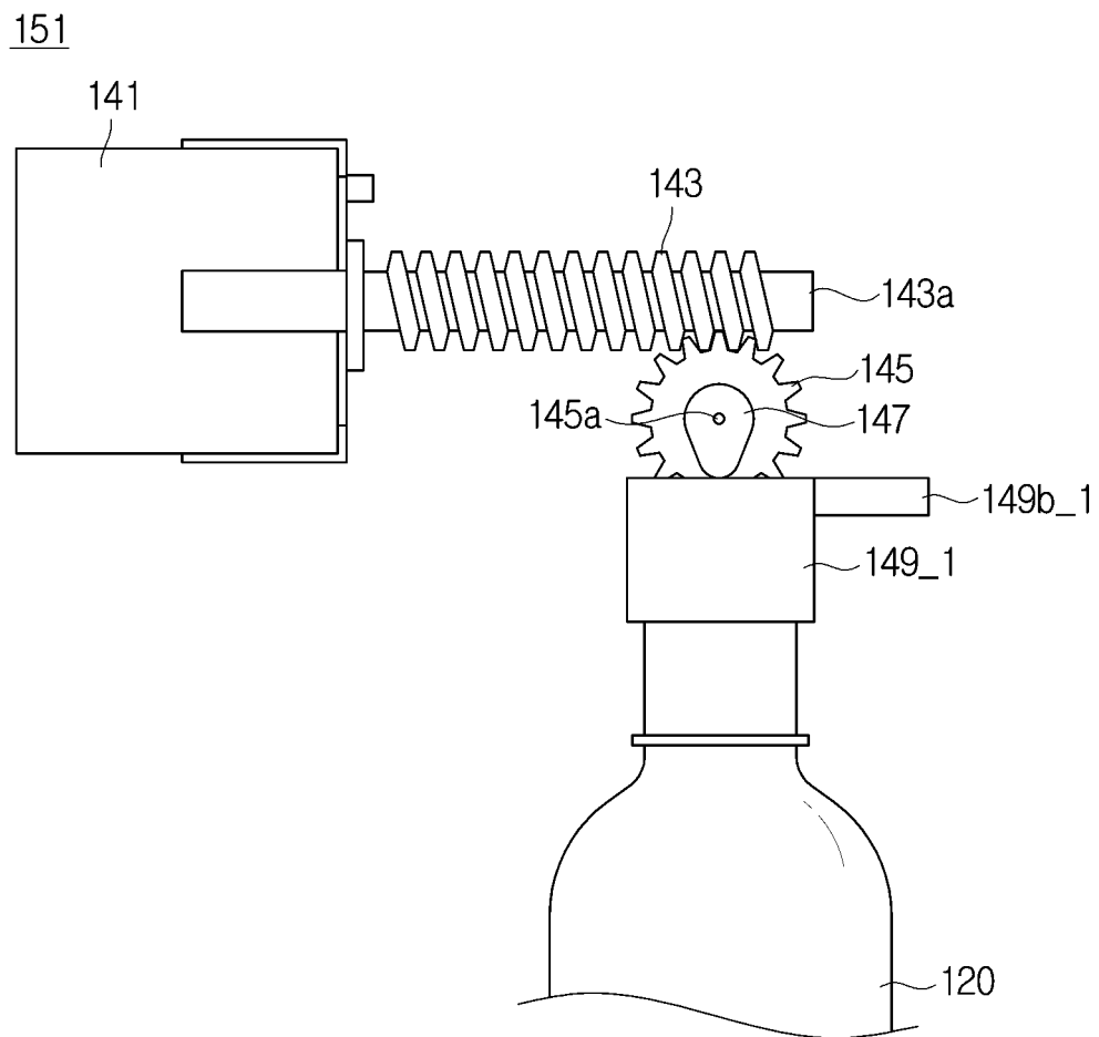
FIG. 7A
