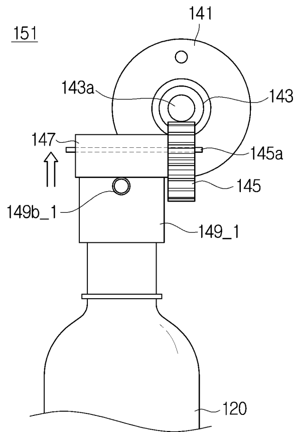
FIG. 7B
