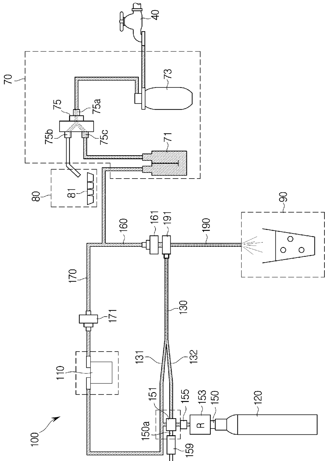
FIG. 11C
