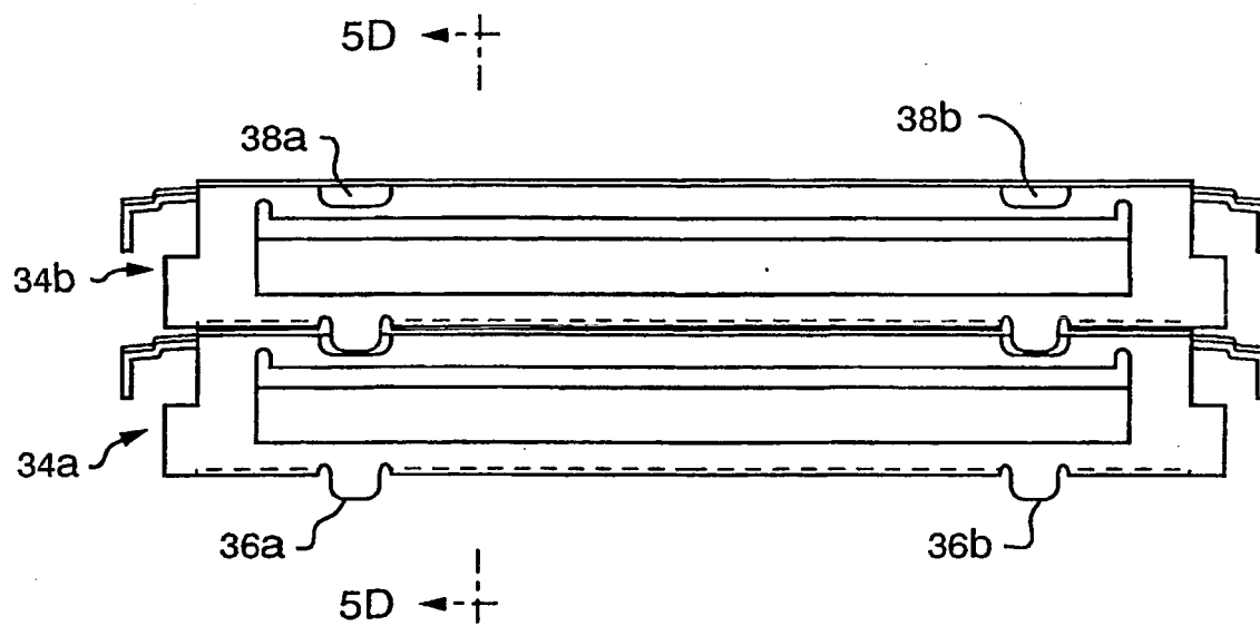
FIG. 5C
