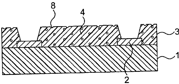
FIG. 4(d) PRIOR ART
