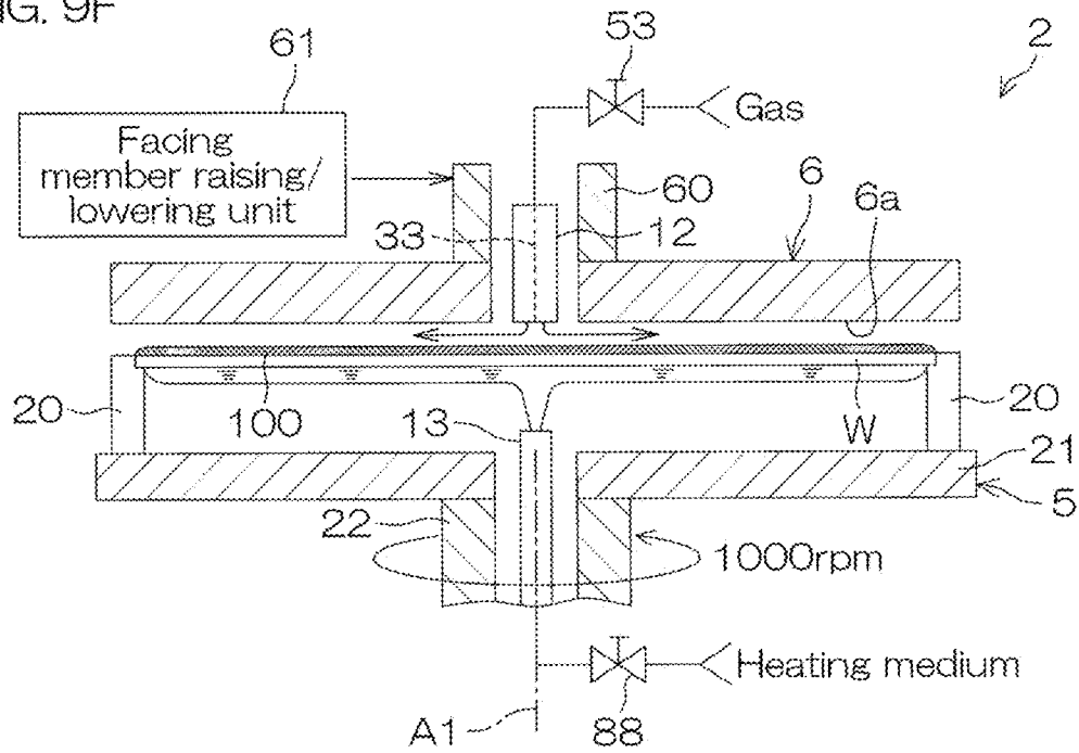
FIG. 9F
