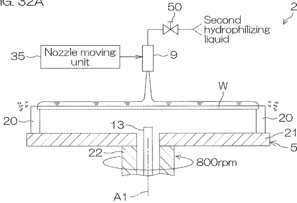
FIG. 32A
