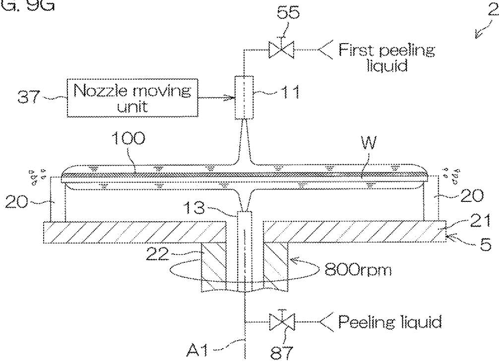
FIG. 9G
