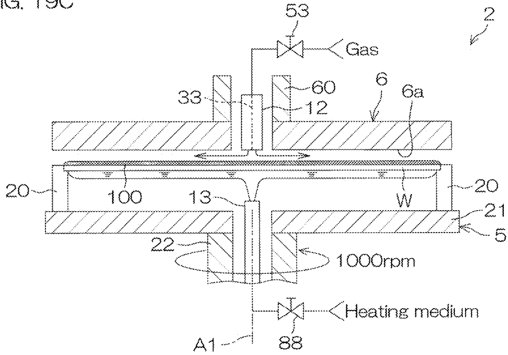
FIG. 19C
