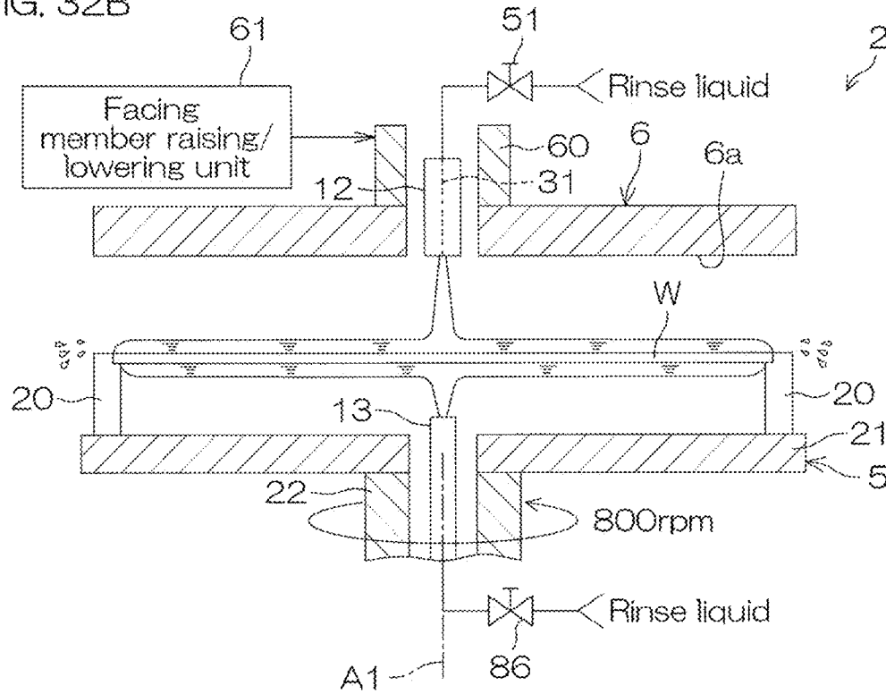
FIG. 32B
