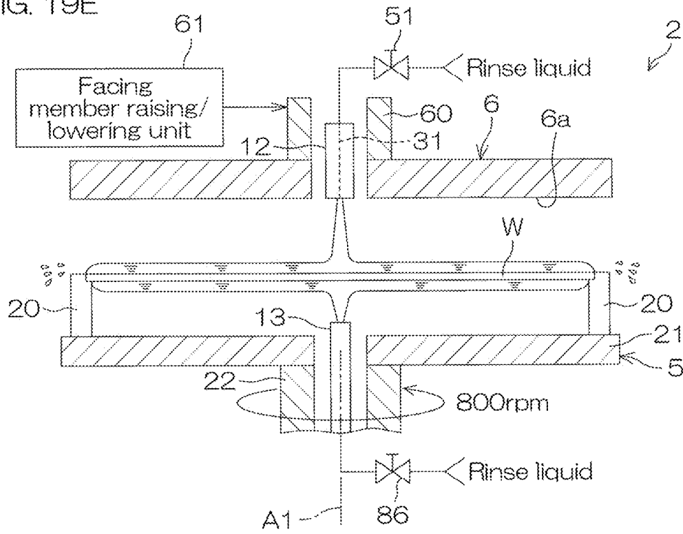
FIG. 19E
