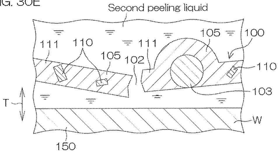
FIG. 30E
