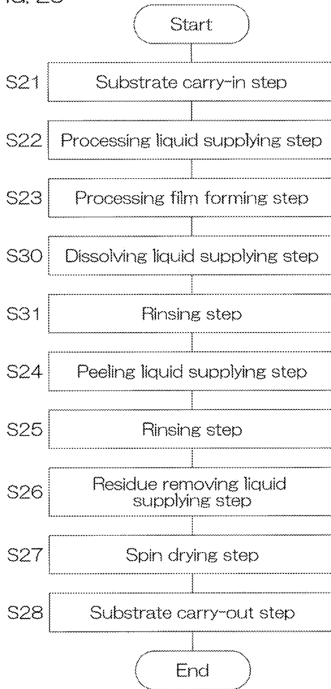
FIG. 23
