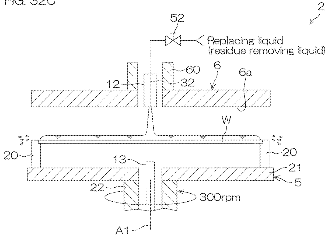
FIG. 32C
