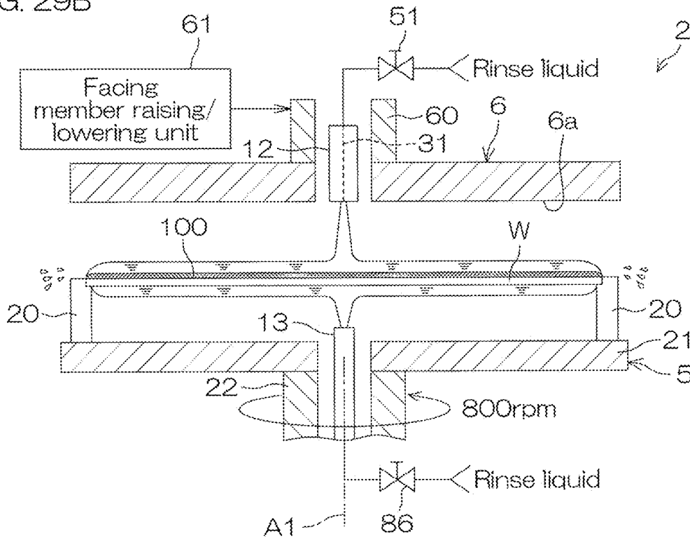
FIG. 29B
