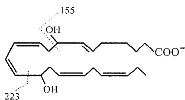
8,14-dihydroxy DPAn-3
