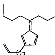
2-(pent-4-enyl)-6,6-dibutylpentafulvene
