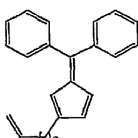
2-(but-3-enyl)-6,6-diphenylpentafulvene
