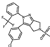
Cpd 15
