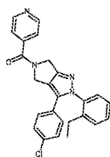
Cpd 5
