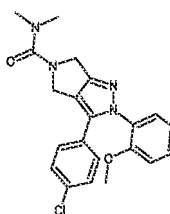
Cpd 34
