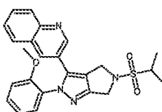
Cpd 93
