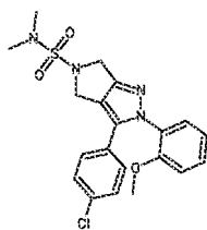
Cpd 33
