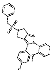
Cpd 39
