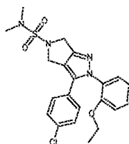
Cpd 54
