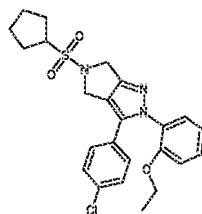
Cpd 51
