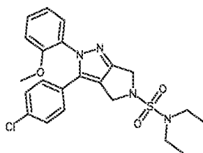
Cpd 56
