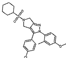
Cpd 68
