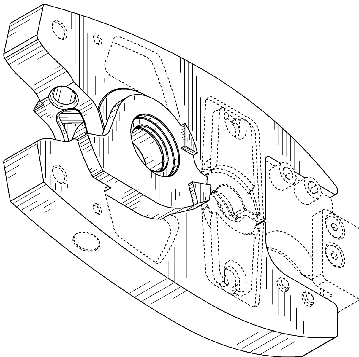
【立體圖3】
