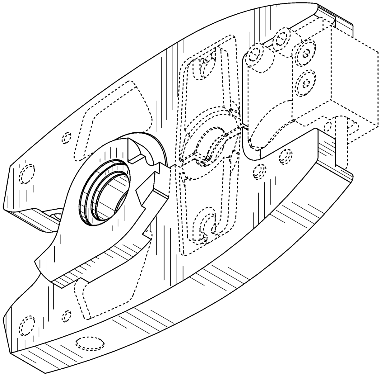
【立體圖4】
