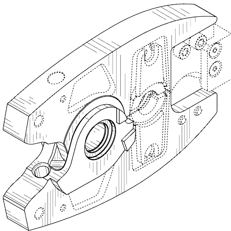
【立體圖1】
