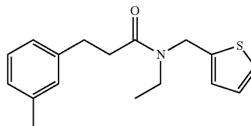
N-ethyl-N-(thiophen-2-ylmethyl)-3-m-tolylpropanamide
