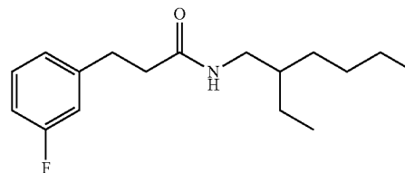
N-(2-ethylhexyl)-3-(3-fluorophenyl)propanamide
