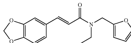
(E)-3-(benzo[d][1,3]dioxol-5-yl)-N-ethyl-N-(furan-2-ylmethyl)acrylamide
