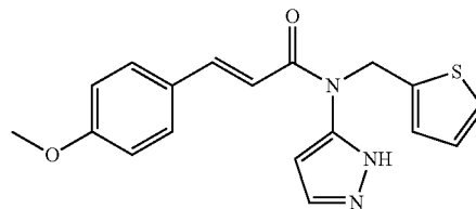
(E)-3-(4-methoxyphenyl)-N-(1H-pyrazol-5-yl)-N-(thiophen-2-ylmethyl)acrylamide
