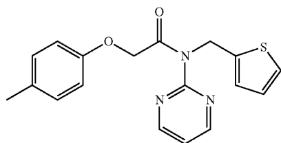
N-(pyrimidin-2-yl)-N-(thiophen-2-ylmethyl)-2-(p-tolyloxy)acetamide
