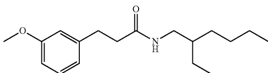
N-(2-ethylhexyl)-3-(3-methoxyphenyl)propanamide
