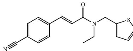
(E)-3-(4-cyanophenyl)-N-ethyl-N-(thiophen-2-ylmethyl)acrylamide
