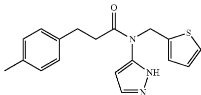
N-(1H-pyrazol-5-yl)-N-(thiophen-2-ylmethyl)-3-p-tolylpropanamide
