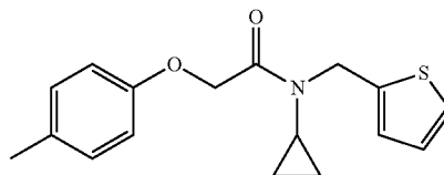
N-cyclopropyl-N-(thiophen-2-ylmethyl)-2-(p-tolyloxy)acetamide
