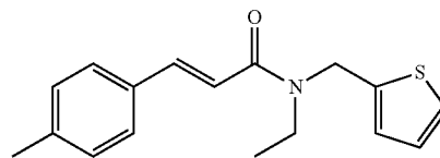
(E)-N-ethyl-N-(thiophen-2-ylmethyl)-3-p-tolylacrylamide
