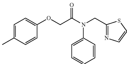
N-phenyl-N-(thiazol-2-ylmethyl)-2-(p-tolyloxy)acetamide
