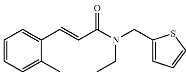
(E)-N-ethyl-N-(thiophen-2-ylmethyl)-3-o-tolylacrylamide
