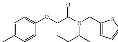
N-sec-butyl-N-(thiophen-2-ylmethyl)-2-(p-tolyloxy)acetamide
