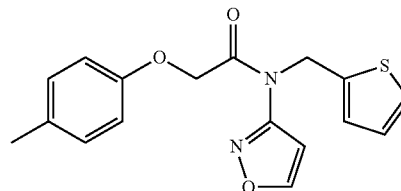
N-(isoxazol-3-yl)-N-(thiophen-2-ylmethyl)-2-(p-tolyloxy)acetamide
