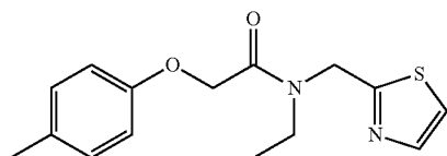
N-ethyl-N-(thiazol-2-ylmethyl)-2-(p-tolyloxy)acetamide
