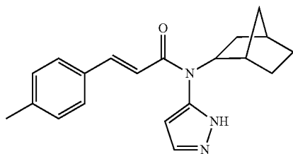
(E)-N-(bicyclo[2.2.1]heptan-2-yl)-N-(1H-pyrazol-5-yl)-3-p-tolylacrylamide
