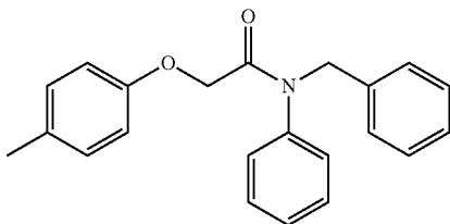
N-benzyl-N-phenyl-2-(p-tolyloxy)acetamide
