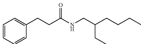
N-(2-ethylhexyl)-3-phenylpropanamide
