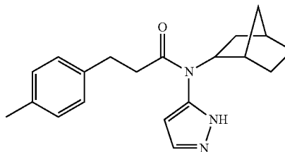
N-(bicyclo[2.2.1]heptan-2-yl)-N-(1H-pyrazol-5-yl)-3-p-tolylpropanamide
