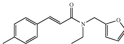
(E)-N-ethyl-N-(furan-2-ylmethyl)-3-p-tolylacrylamide
