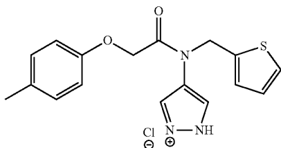
4-(N-(thiophen-2-ylmethyl)-2-(p-tolyloxy)acetamido)-1H-pyrazol-2-ium chloride
