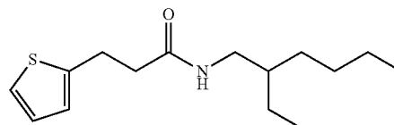
N-(2-ethylhexyl)-3-(thiophen-2-yl)propanamide
