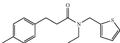
N-ethyl-N-(thiophen-2-ylmethyl)-3-p-tolylpropanamide
