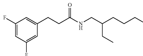
3-(3,5-difluorophenyl)-N-(2-ethylhexyl)propanamide
