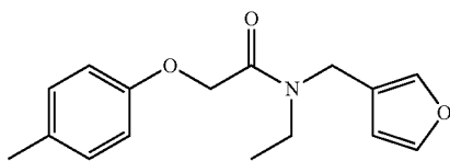
N-ethyl-N-(furan-3-ylmethyl)-2-(p-tolyloxy)acetamide
