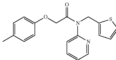
N-(pyridin-2-yl)-N-(thiophen-2-ylmethyl)-2-(p-tolyloxy)acetamide
