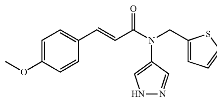
(E)-3-(4-methoxyphenyl)-N-(1H-pyrazol-4-yl)-N-(thiophen-2-ylmethyl)acrylamide
