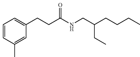
N-(2-ethylhexyl)-3-m-tolylpropanamide
