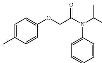
N-isopropyl-N-phenyl-2-(p-tolyloxy)acetamide
