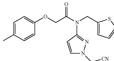
N-(1-(cyanomethyl)-1H-pyrazol-3-yl)-N-(thiophen-2-ylmethyl)-2-(p-tolyloxy)acetamide
