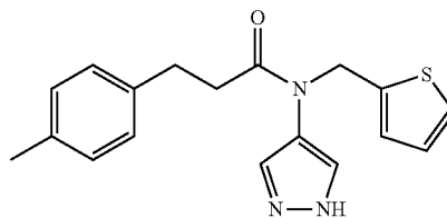
N-(1H-pyrazol-4-yl)-N-(thiophen-2-ylmethyl)-3-p-tolylpropanamide
