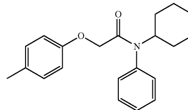
N-cyclohexyl-N-phenyl-2-(p-tolyloxy)acetamide
