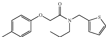
N-propyl-N-(thiophen-2-ylmethyl)-2-(p-tolyloxy)acetamide
