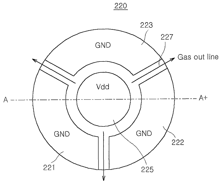
2/3 FIG. 3
