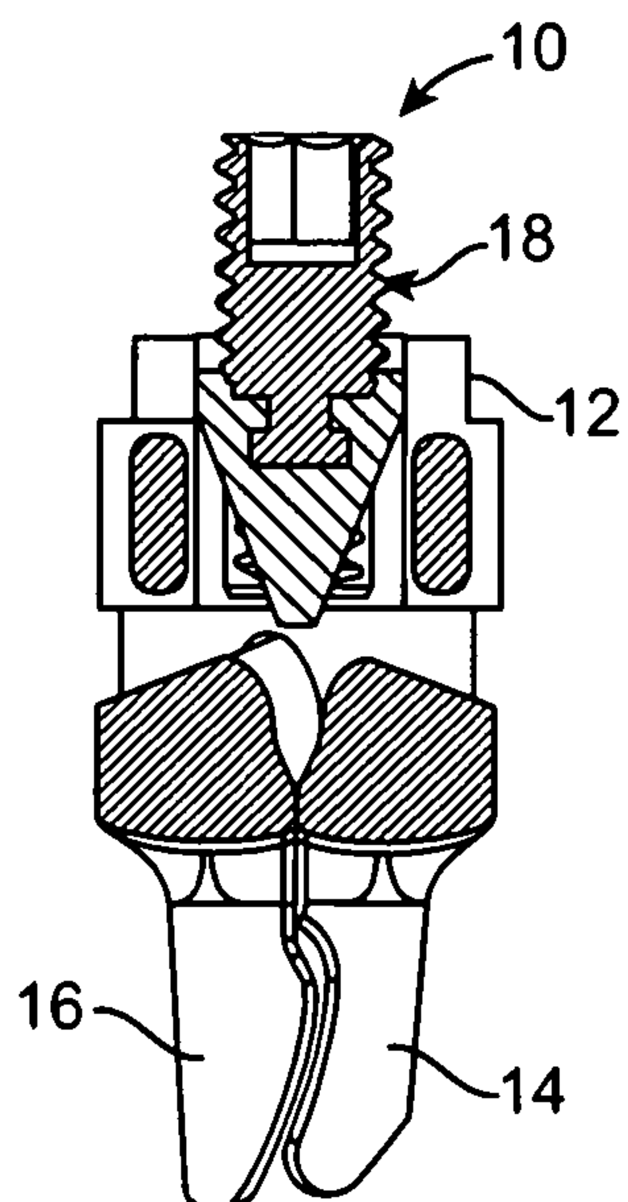
SECTION A-A
