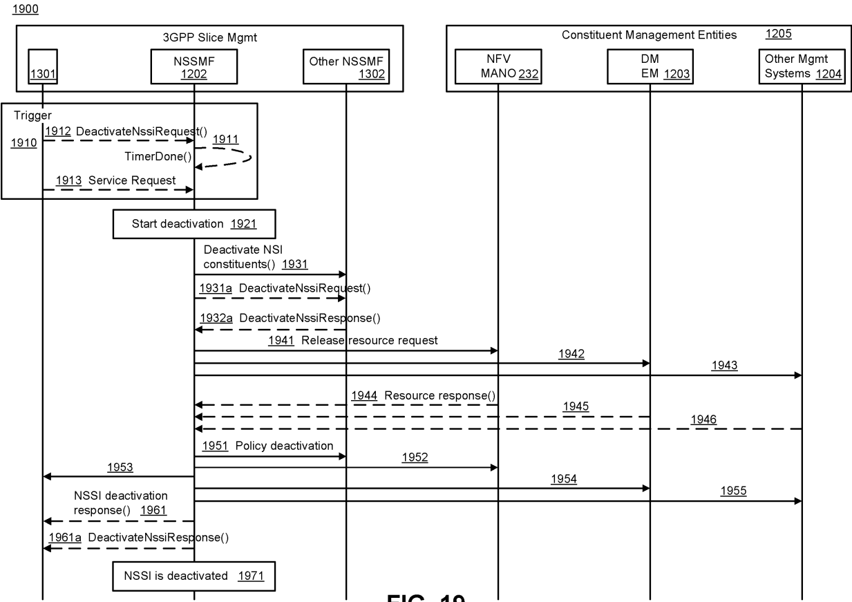
FIG. 19
