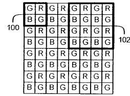
FIG. 2 (従来技術)
