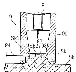
FIG.18C 従来技術
