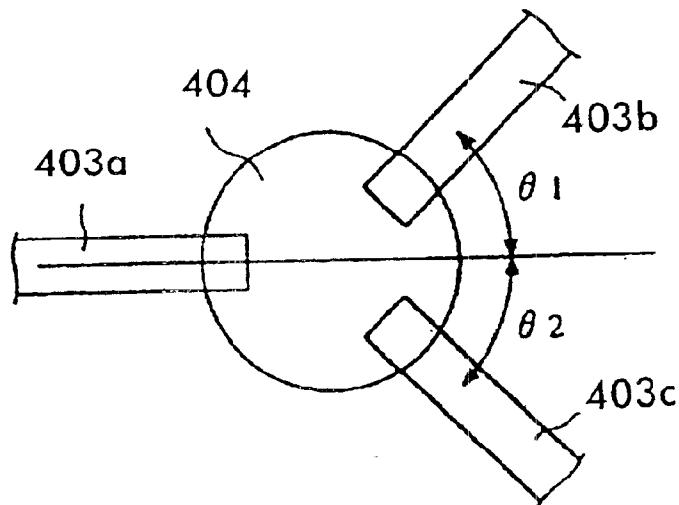
FIG. 13C
