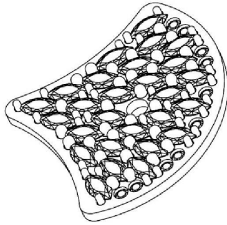
【立體圖 1】
